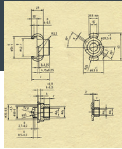
Technische Zeichnung
